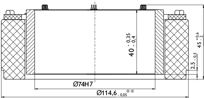
Эскиз с присоединительными размерами
