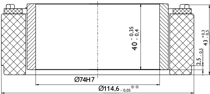
Эскиз с присоединительными размерами
