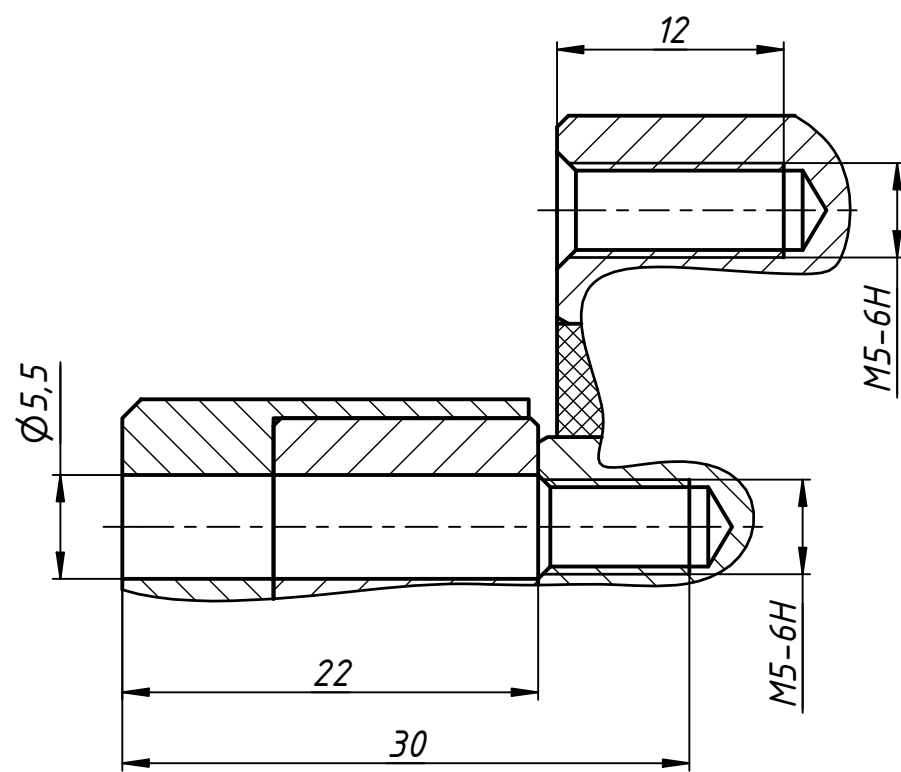
A-A (2,5:1) \odot 16 мест
