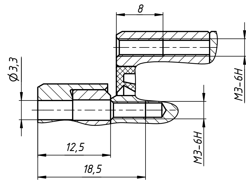
A-A (2,5 : 1) \odot 16 мест
