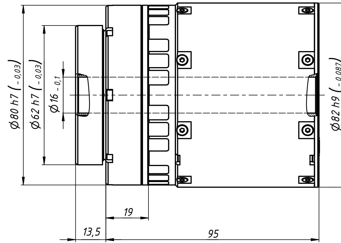
Б (4 : 1)
