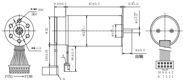
不带减速箱外形图 (Motor without gearbox)
