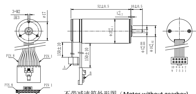
不带减速箱外形图 (Motor without gearbox)
